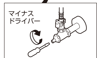
図4 止水栓での流量調節
