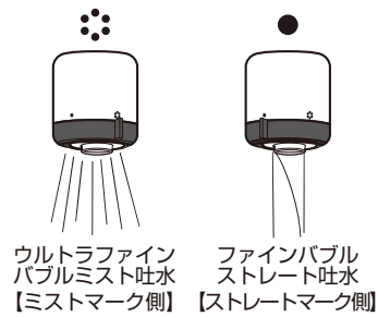
図5 吐出切替
