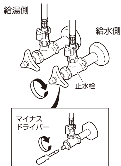
図6 給水側バルブ操作
